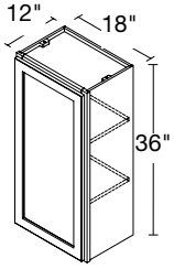
1 DOOR 18" | W1836(L/R)
