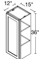
1 DOOR 15" | W1536(L/R)
