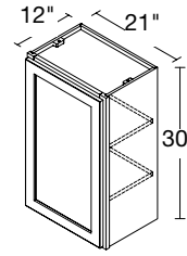
1 DOOR 21" | W2130(L/R)
