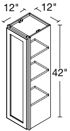
1 DOOR 12" | W1242(L/R)
