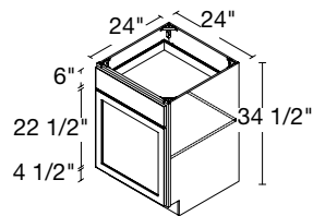
1 DOOR / 1 DRAWER 24" | B24(L/R)
