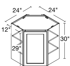
1 DOOR WALL CORNER 24" | WA2430(L/R)
