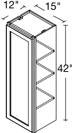
1 DOOR 15" | W1542(L/R)
