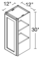
1 DOOR 12" | W1230(L/R)
