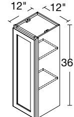
1 DOOR 12" | W1236(L/R)
