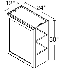
1 DOOR 24" | W2430(L/R)
