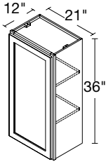
1 DOOR 21" | W2136(L/R)
