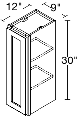
1 DOOR 9" | W930(L/R)
