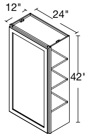
1 DOOR 24" | W2442(L/R)
