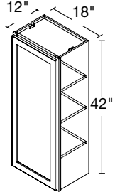
1 DOOR 18" | W1842(L/R)
