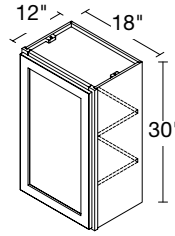
1 DOOR 18" | W1830(L/R)
