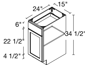
1 DOOR / 1 DRAWER 15" | B15(L/R)
