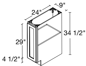
1 DOOR 9" | B9FH(L/R)
