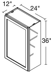
1 DOOR 24" | W2436(L/R)
