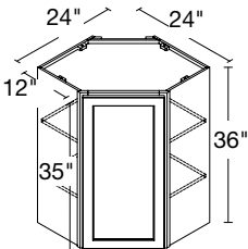
1 DOOR WALL CORNER 24" | WA2436(L/R)
