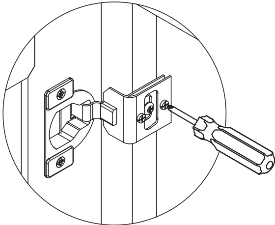
Réglage avant/arrière
