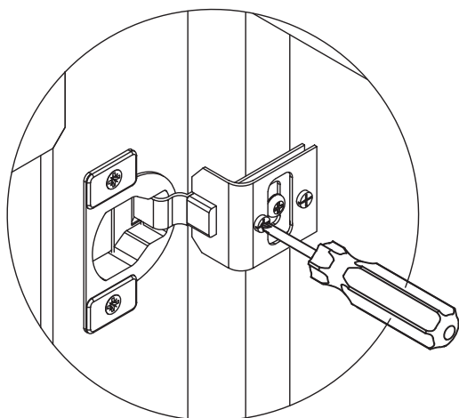
Réglage gauche/droite
